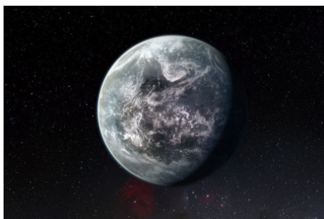
6-сурет – Ғаламшар
