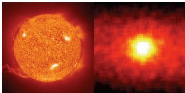
10-сурет – Нейтрино
